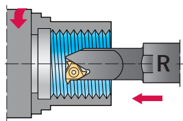
Правая резьба правая державка правая пластина
