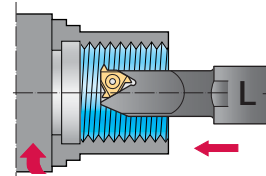
Левая резьба левая державка левая пластина
